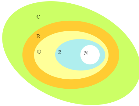
1.5. ábra. Számhalmazok
